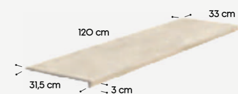
Peldaño recto 120 33 x 120 x 3 cm 13.0" x 47.2" x 1.2"
